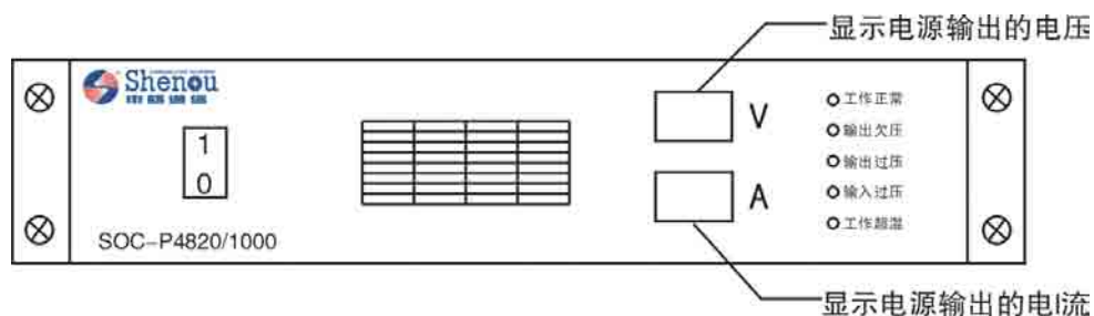
图 3-21 SOC-P4820/1000 电源箱前面板示意图
