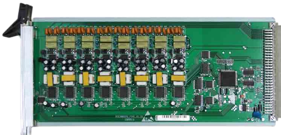
图 3-16 FXS 用户板
