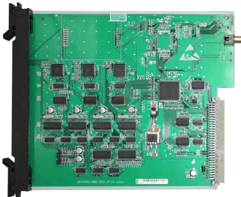
图 3-4 SCU 分控板
