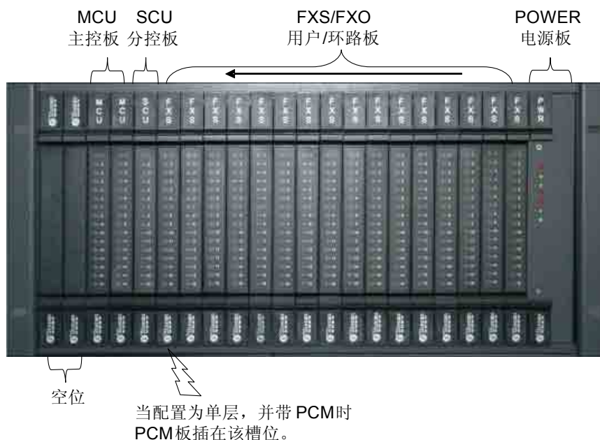
图 3-2 主机框
