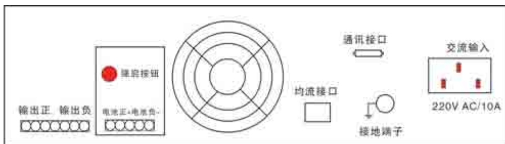
图 3-9 SOC-P4820/1000 电源箱背面板示意图
