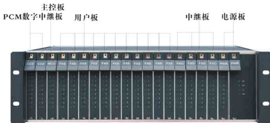
图 3-13 JSY2000-06S 机框的正面
