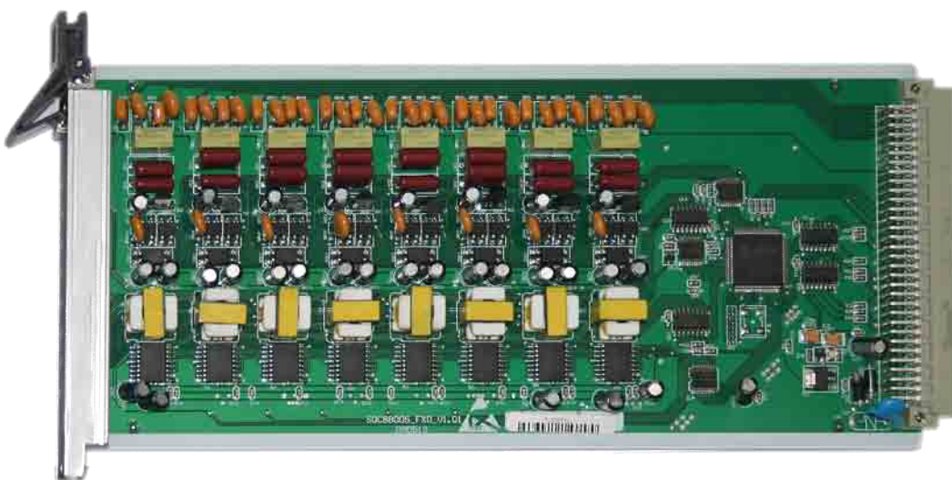
图 3-17 FXO 环路中继板
