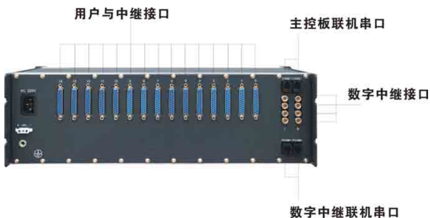
图 3-14 JSY2000-06S 机框的背面
