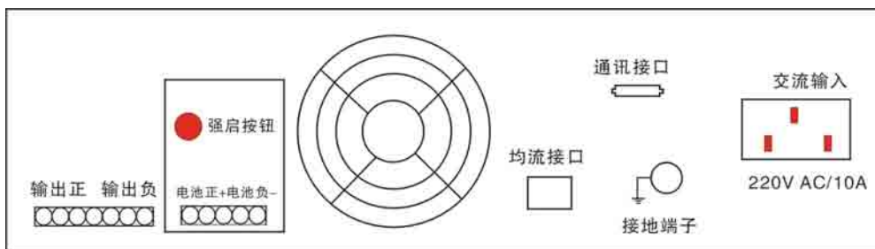
图 3-22 SOC-P4820/1000 电源箱背面板示意图
