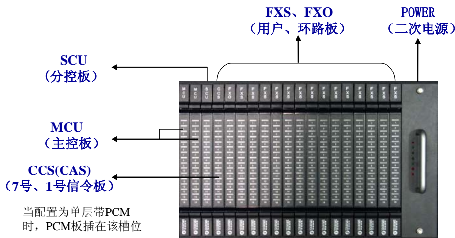
图 3-3 主框示意图
